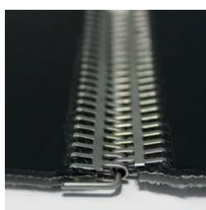
Giunzione metallica annegata
